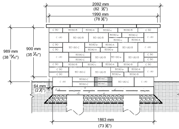
ELEVATION A
